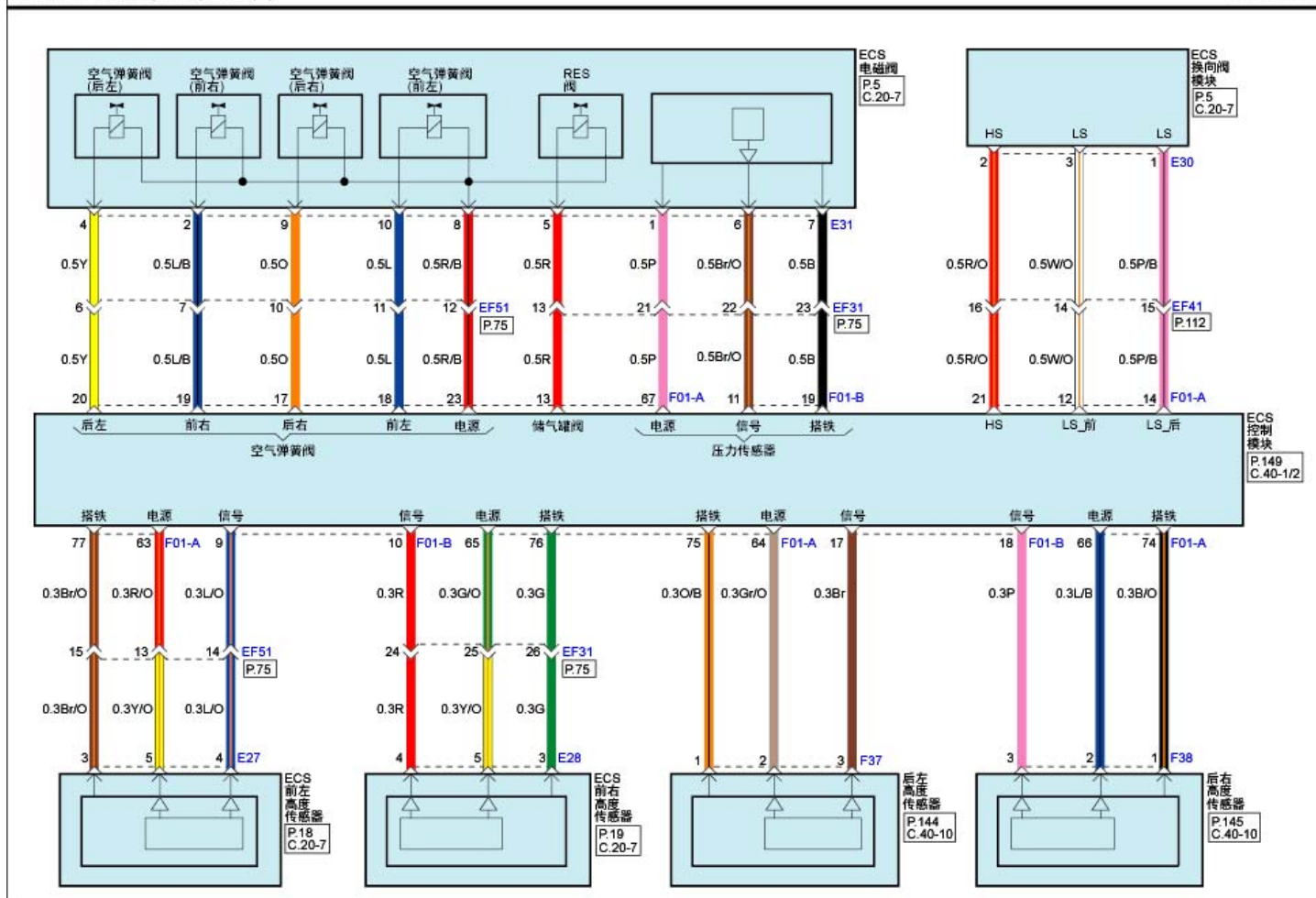
电控空气悬架(EAS)系统(2)
